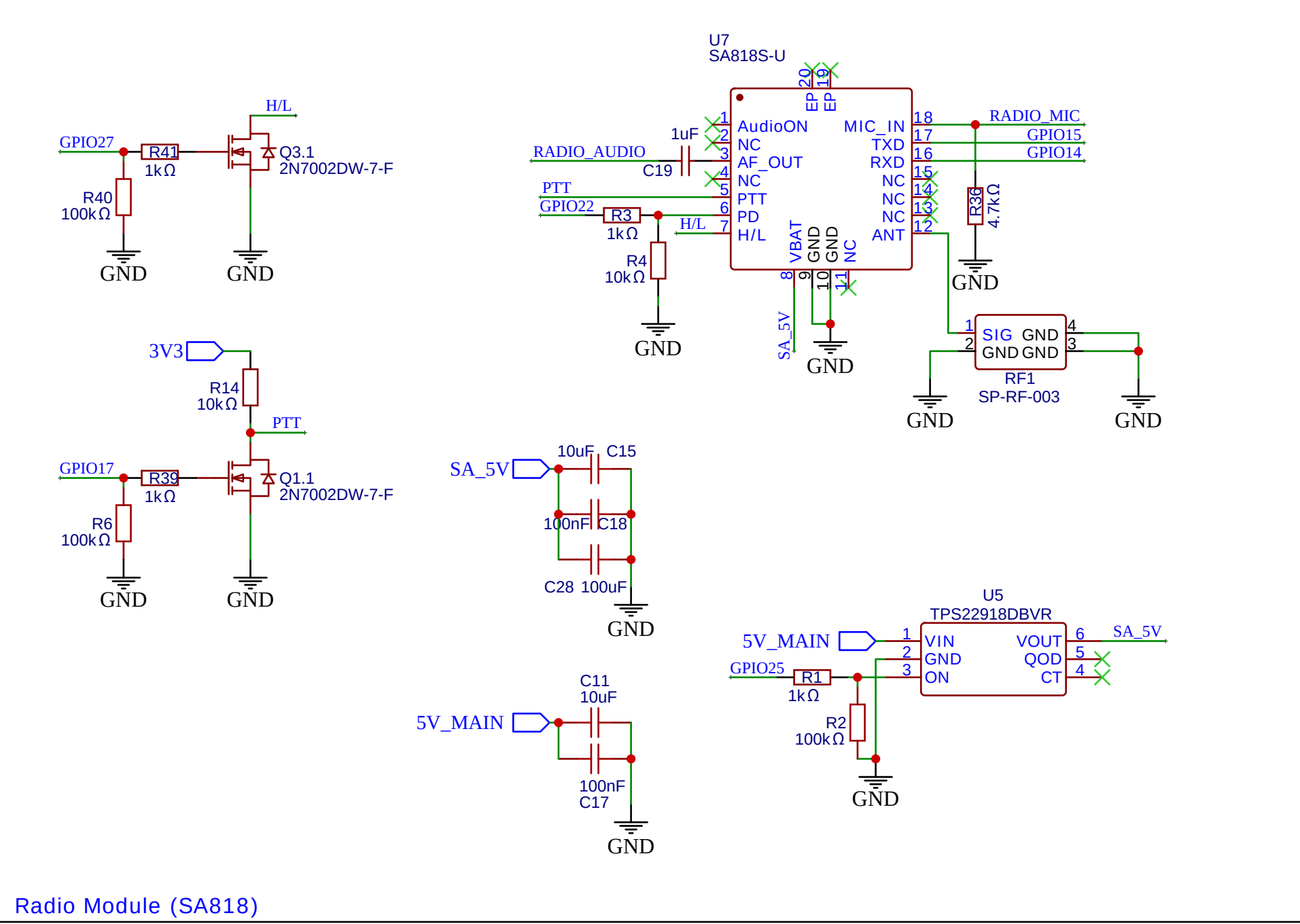
Radio Module (SA818)
